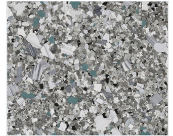
Turquoise
